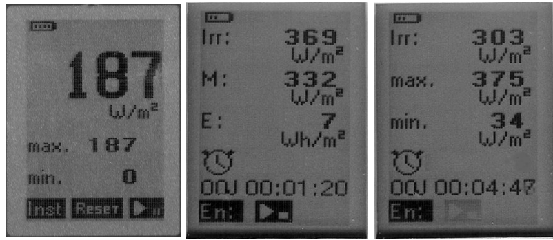
Eclairage énergétique Valeurs Max, Min Irradiation, moyenne, énergie cumulée, Max et Min de l'irradiation instantanée
