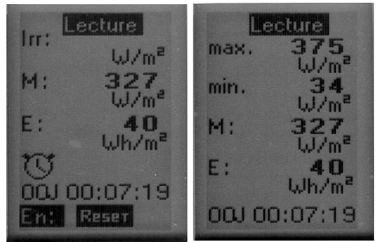
Irradiation, moyenne, énergie cumulée, Max et Min de l'irradiation instantanée
